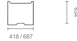
FMQ10.04/11.06 418 × 85 × 634 / 687 × 85 × 634
