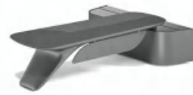
MLG80L.32/MLG80L.28/MLG80L.24 3200*2400*760/2800*2400*760/2400*2100*760 (mm)
