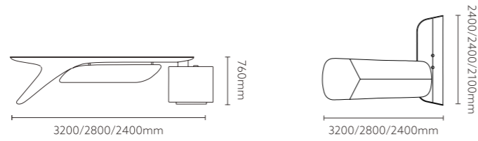
MLG80L.32/MLG80L.28/MLG80L.24 3200*2400*760/2800*2400*760/2400*2100*760 (mm)
