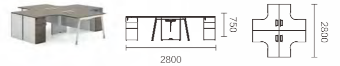
FNQ57.28BJ 2800 × 2800 × 750
