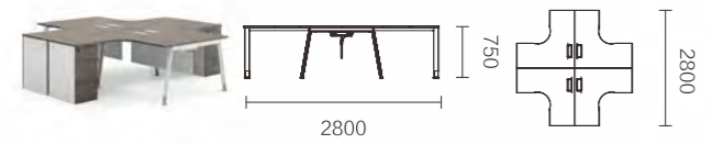
FNQ56.28BJ 2800 × 2800 × 750
