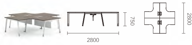
FNQ54.28BJ 2800 × 2800 × 750
