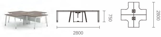
FNQ55.28BJ 2800 × 2800 × 750
